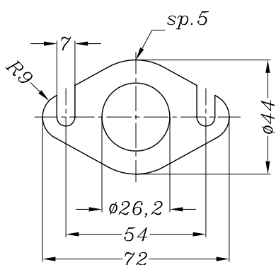
Vista da "A" Flangia tipo "99A"
