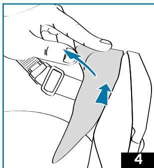
4 - Každou lícnici zcela vyjměte zevnitř přilby přesunutím přes konec podbradního pásku; v případě potřeby přilbu otočte.
